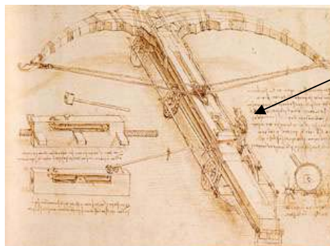
Ontwerpschets van een grote kruisboog door Leonardo da Vinci (bron: Bibliotheca Ambrosiana, Italië ). Om een beeld te krijgen van de omvang van de kruisboog: de zwarte pijl wijst naar de man die het gevaarte bediend.
